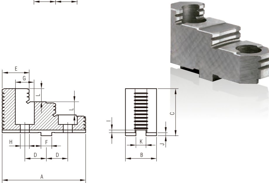
GARRA PARTIDA ALTA DURA HARD TOP JAW
