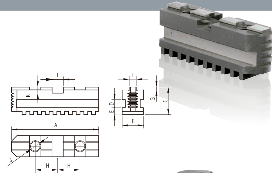
GARRAS PARTIDAS BASE HARD MASTER JAW
