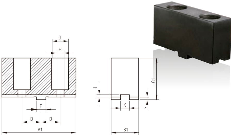
GARRA PARTIDA ALTA BLANDA SOFT TOP JAW
