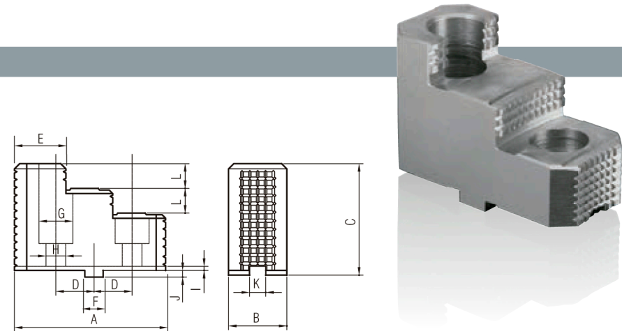
GARRA PARTIDA ALTA DURA HARD TOP JAWS - Las garras de los platos 1250,1400,1600 y 2000 tienen una escalera - The jaws for chucks diam.1250,1400,1600 and 2000 goes just with one step.
