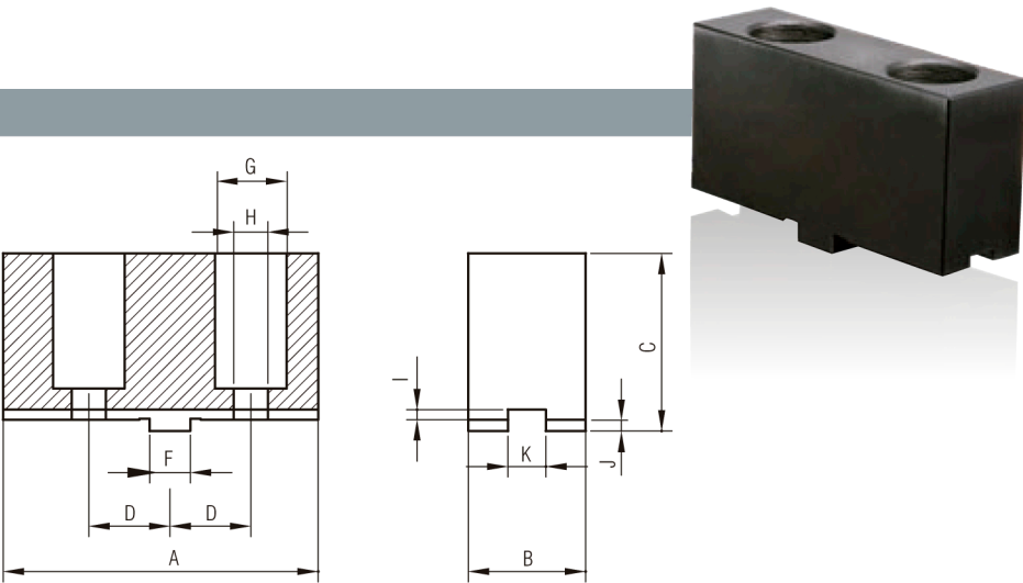
GARRA PARTIDA ALTA BLANDA SOFT TOP JAW
